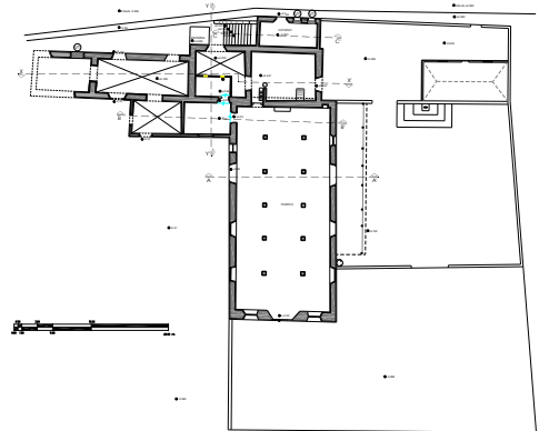
PLANTA ARQUITECTÓNICA
