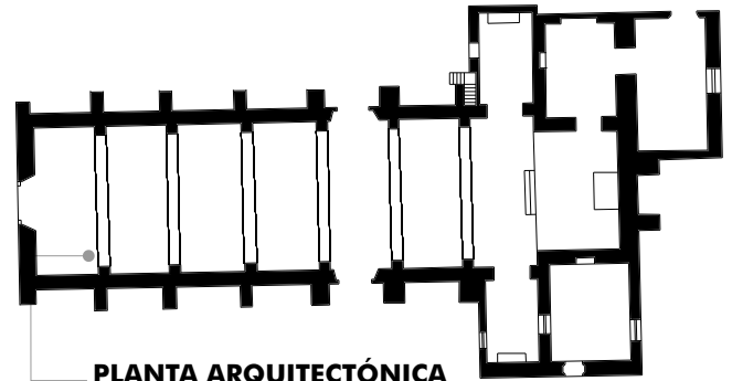
PLANTA ARQUITECTÓNICA
