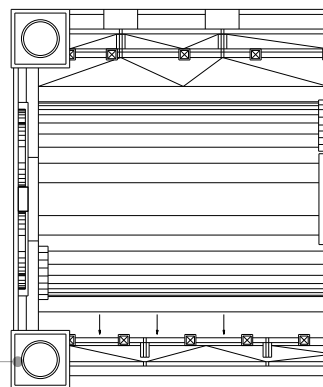
PLANTA DE AZOTEA
